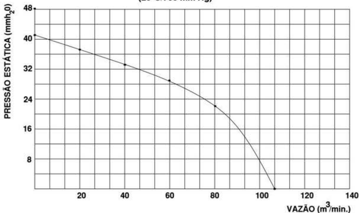
CURVA CARACTERÍSTICA (20°C/760 mm Hg)
