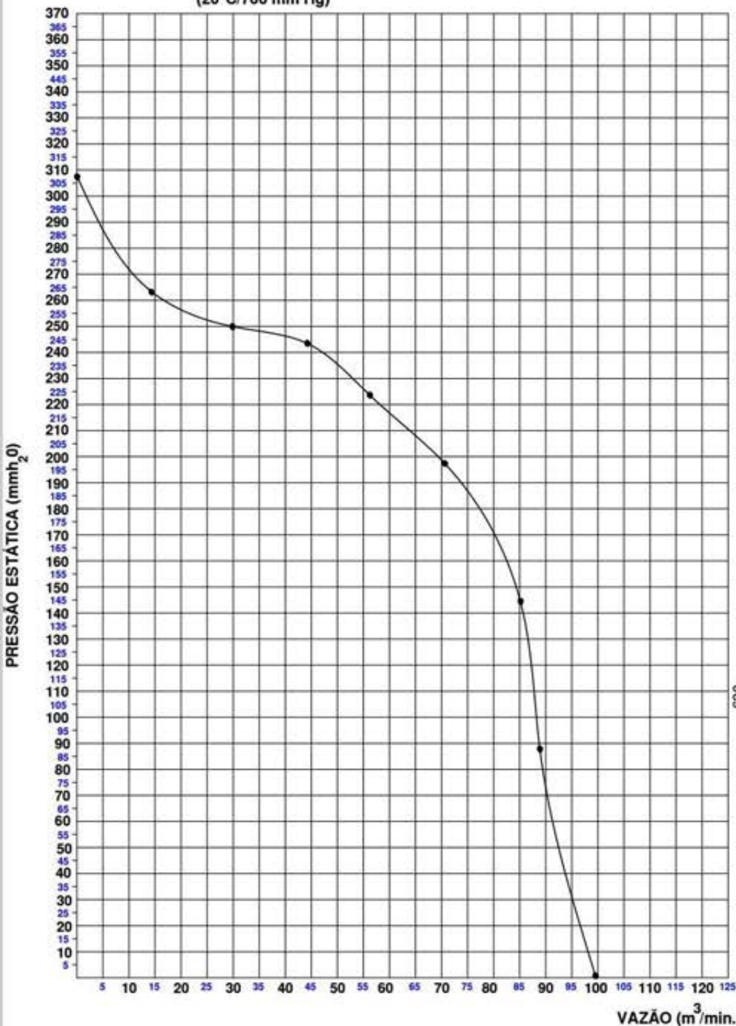
CURVA CARACTERÍSTICA (20°C/760 mm Hg)
